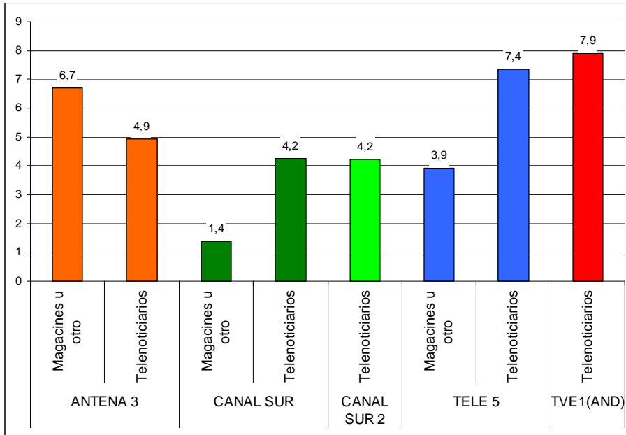
Gráfico 13: Índice de impacto, escenas de violencia. Media: 4,5
