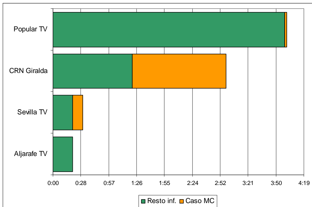
Gráfico 5: Desglose de tiempos cadenas locales (valores absolutos en horas)
