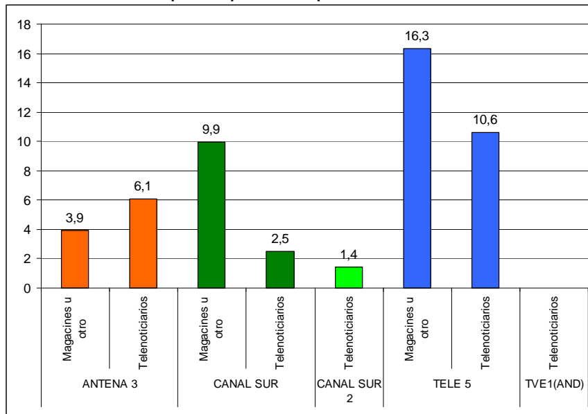
Gráfico 8: Índice de impacto, aparición de posibles menores. Media: 8,4
