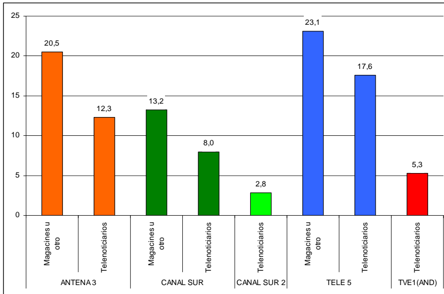
Gráfico 12: Índice de impacto, testimonios circunstanciales. Media: 15,8
