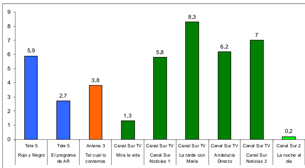
Gráfico 2: Índices de audiencia de los programas seleccionados para el estudio cualitativo (audiencia %)
