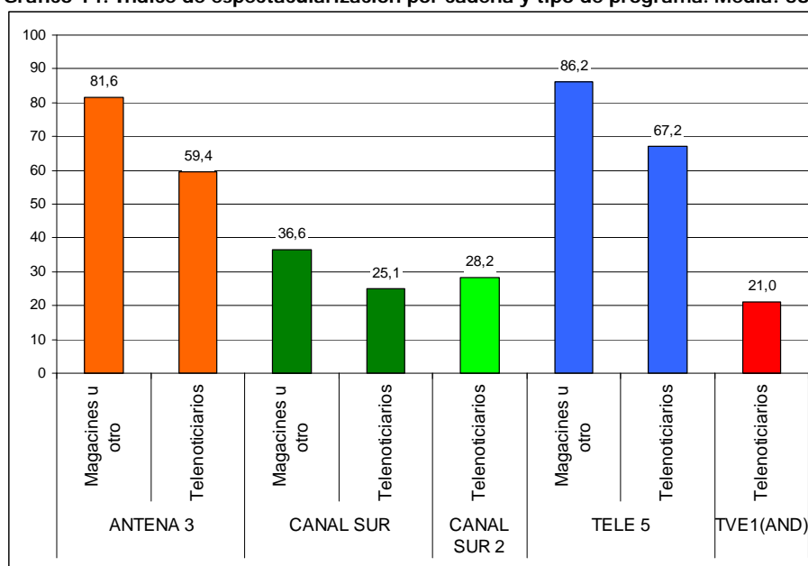
Gráfico 14: Índice de espectacularización por cadena y tipo de programa. Media: 58,6
