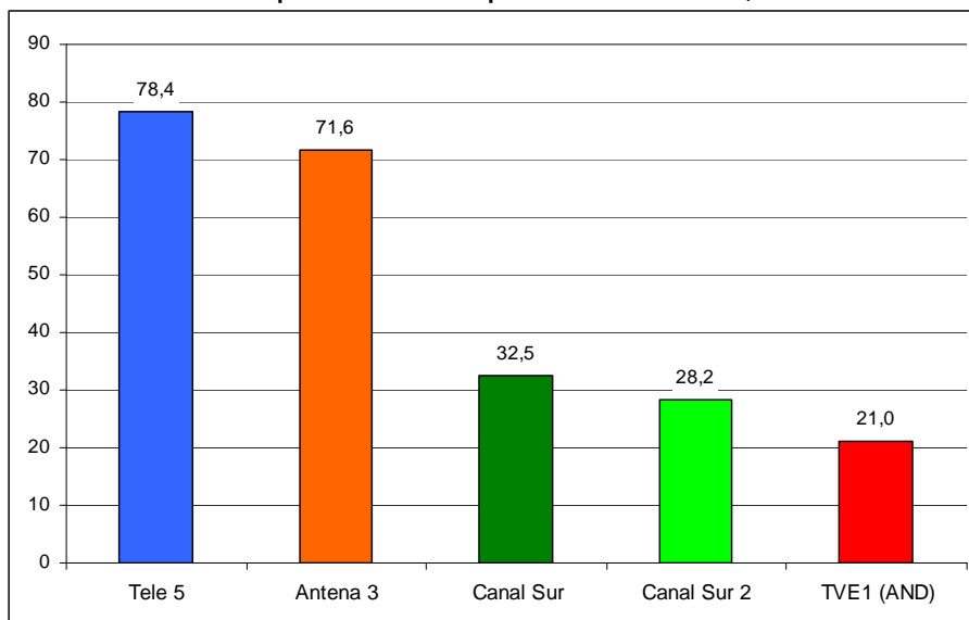
Gráfico 15: Índice de espectacularización por cadena. Media: 58,6
