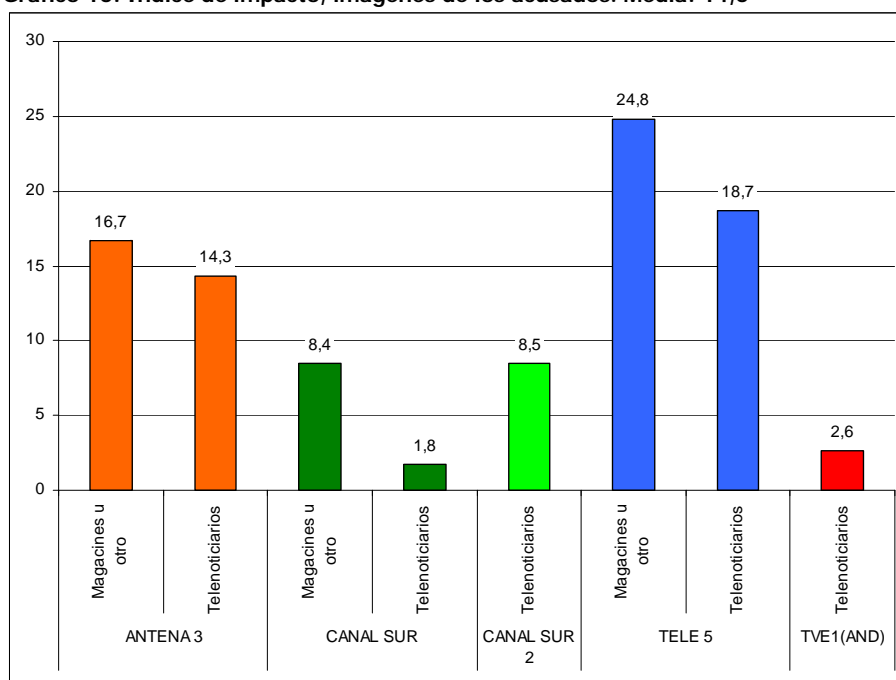
Gráfico 10: Índice de impacto, imágenes de los acusados. Media: 14,0
