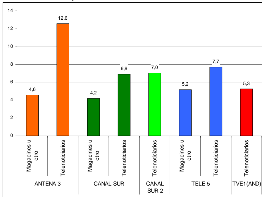
Gráfico 9: Índice de impacto, escenas de duelo. Media: 6,5
