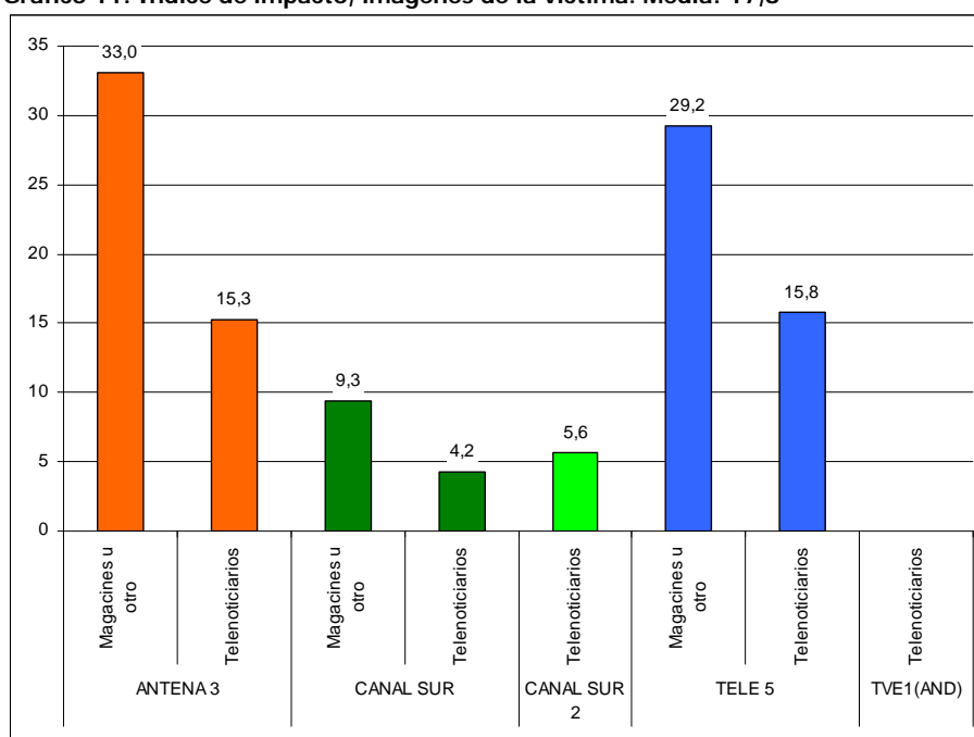
Gráfico 11: Índice de impacto, imágenes de la víctima. Media: 17,8
