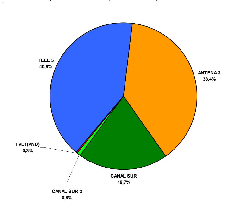
Gráfico 7: Porcentaje de indicadores de espectacularización por cadenas.
